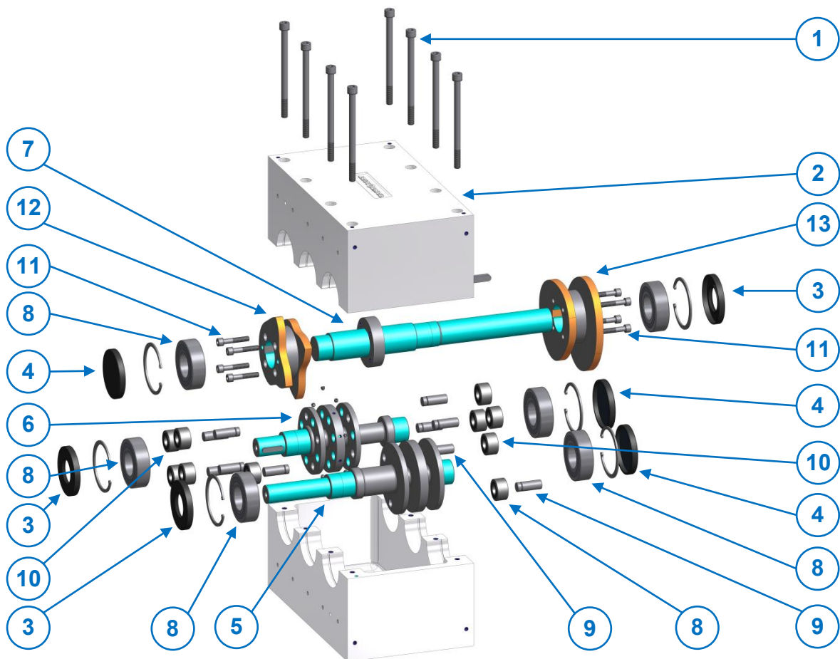
Abb. 38 Detail Montager Reihenfolge SP105
