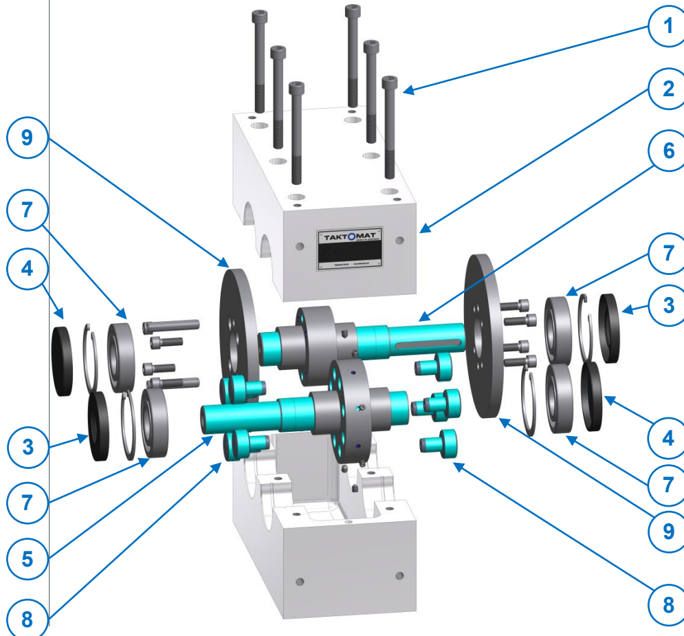
Abb. 35 Detail Montagereihenfolge TP040-100 / XP030-130
