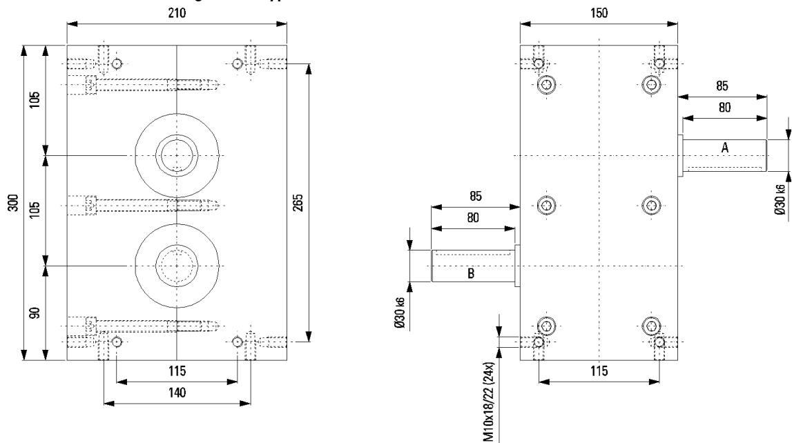
Abb. 16 Maßzeichnung XP 105
