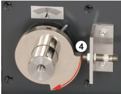
Abb. 33 Detail Zeitverzögertes Abschalten
