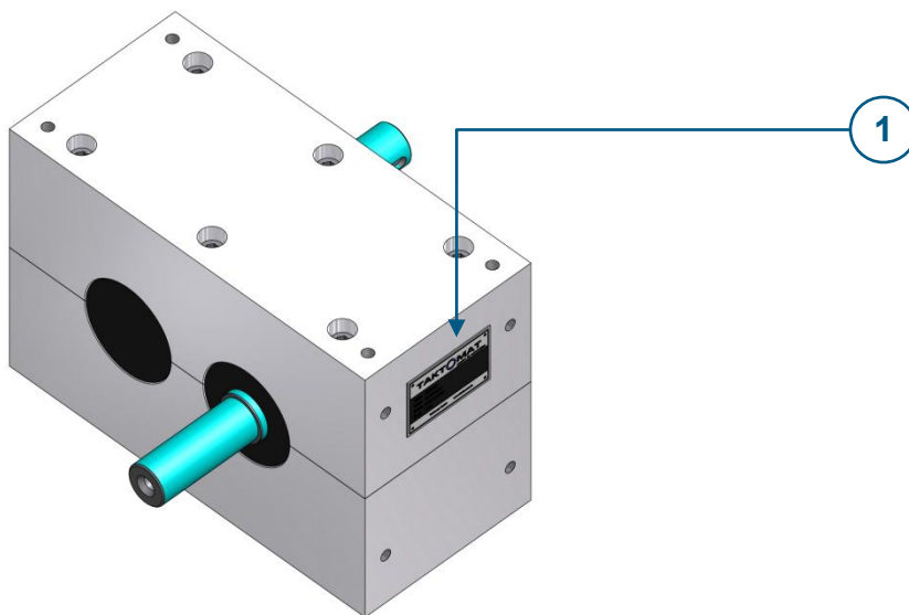
Abb. 3 Position Typenschild
