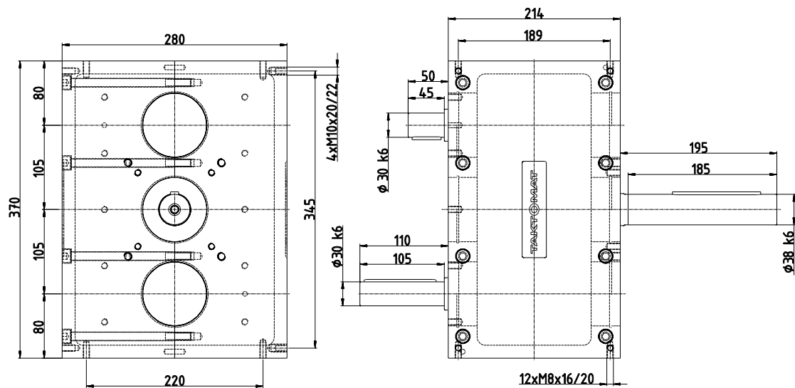
Abb. 27 Maßzeichnung SP 105
