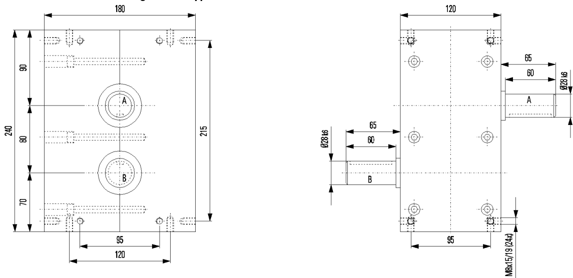
Abb. 15 Maßzeichnung XP 080
