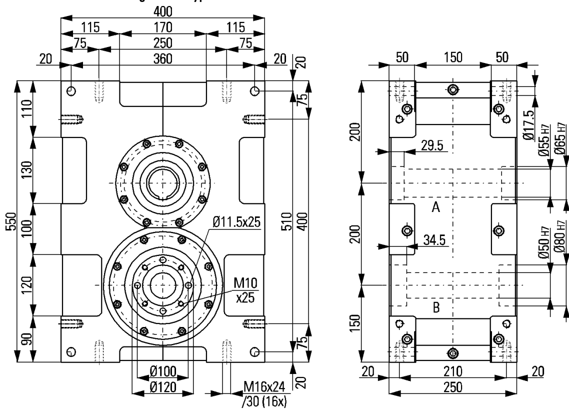
Abb. 19 Maßzeichnung XP 200
