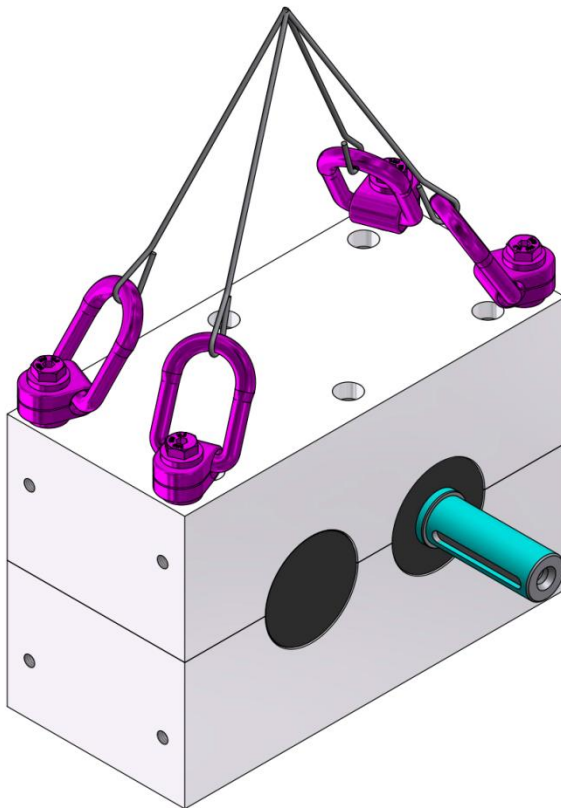
Abb. 28 Transport mit Ringschrauben
