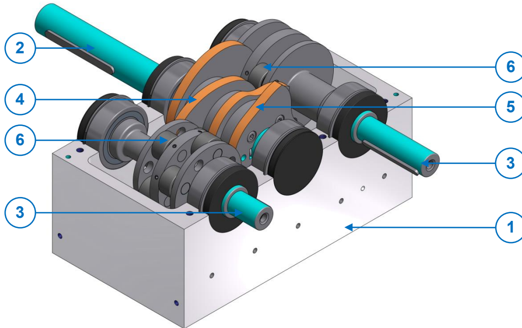
Abb. 9 Aufbau Scheibenkurven-Schrittgetriebe SP
