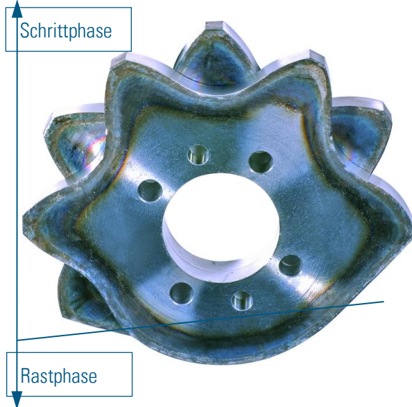
Abb. 10 Scheibenkurvensatz Rast – und Schaltphase
