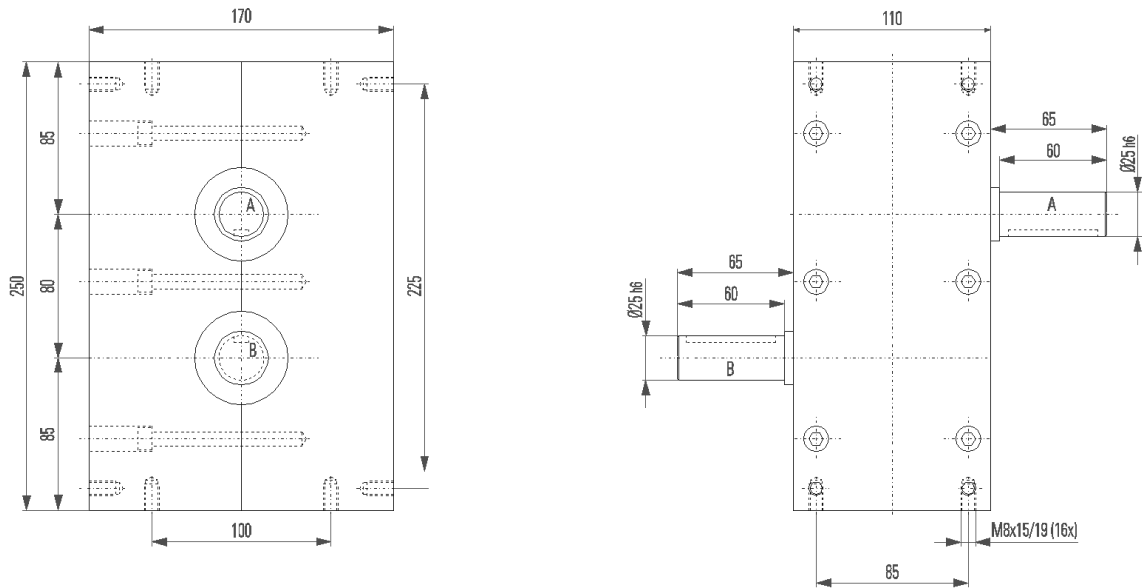
Abb. 23 Maßzeichnung TP 080
