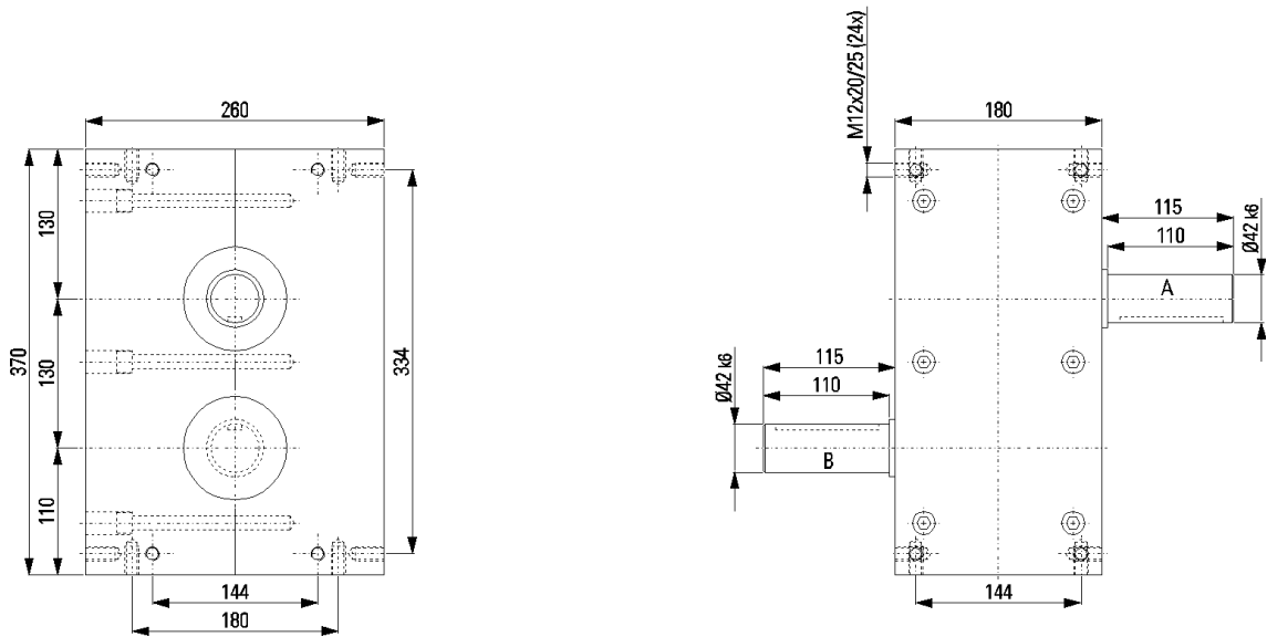
Abb. 17 Maßzeichnung XP 130
