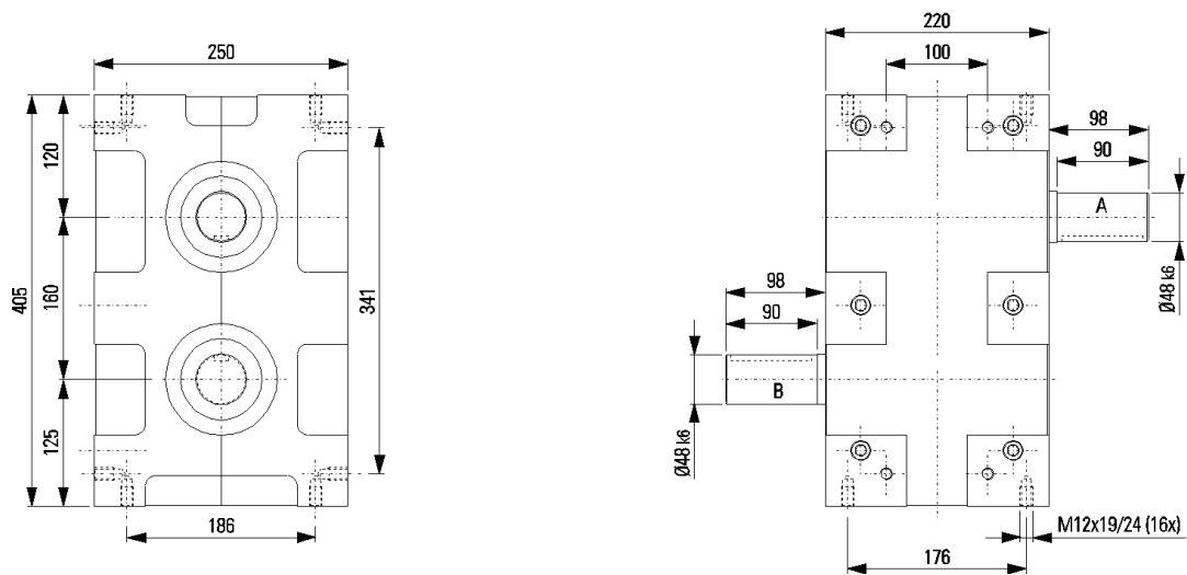
Abb. 26 Maßzeichnung TP 160
