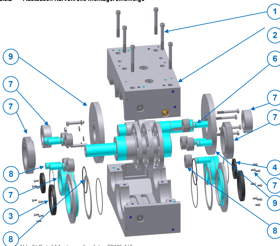
Abb. 36 Detail Montager Reihenfolge TP125-160
