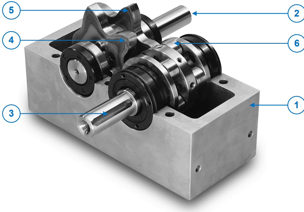
Abb. 4 Aufbau Scheibenkurven-Schrittgetriebe XP - TP – SP
