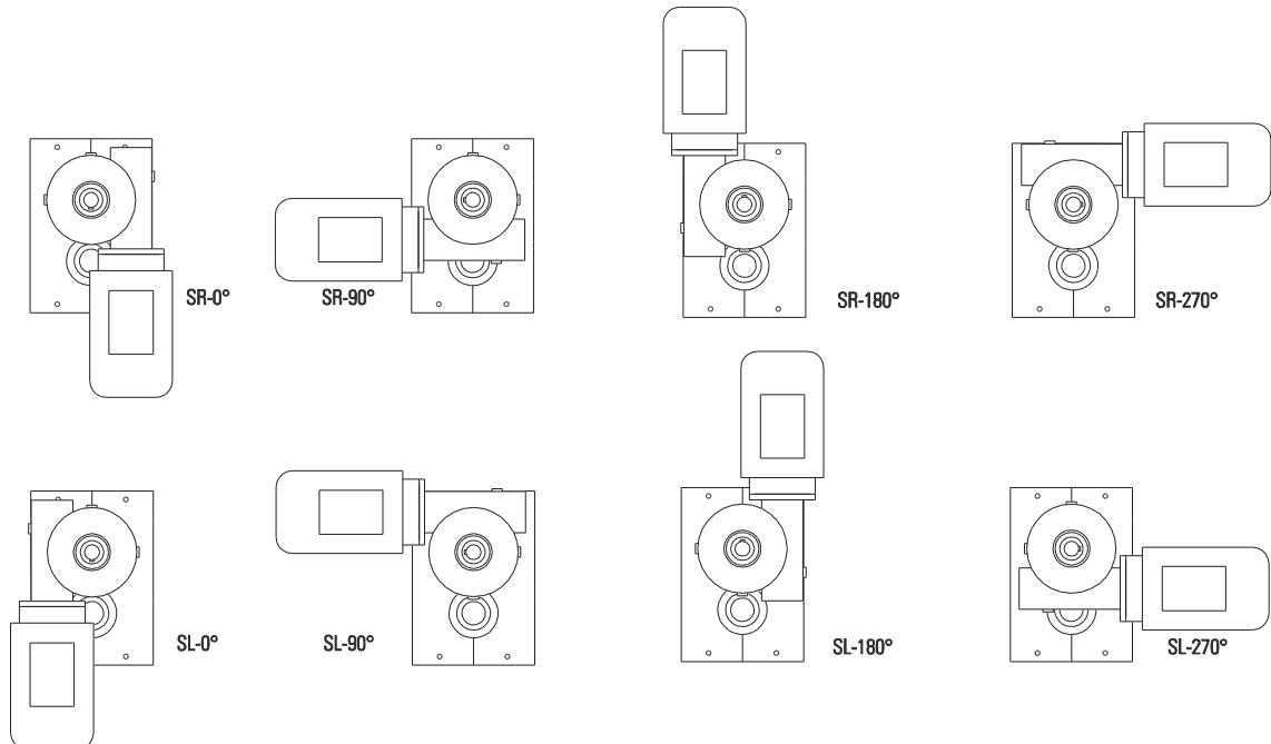
Abb. 30 Anbautagen Antrieb
