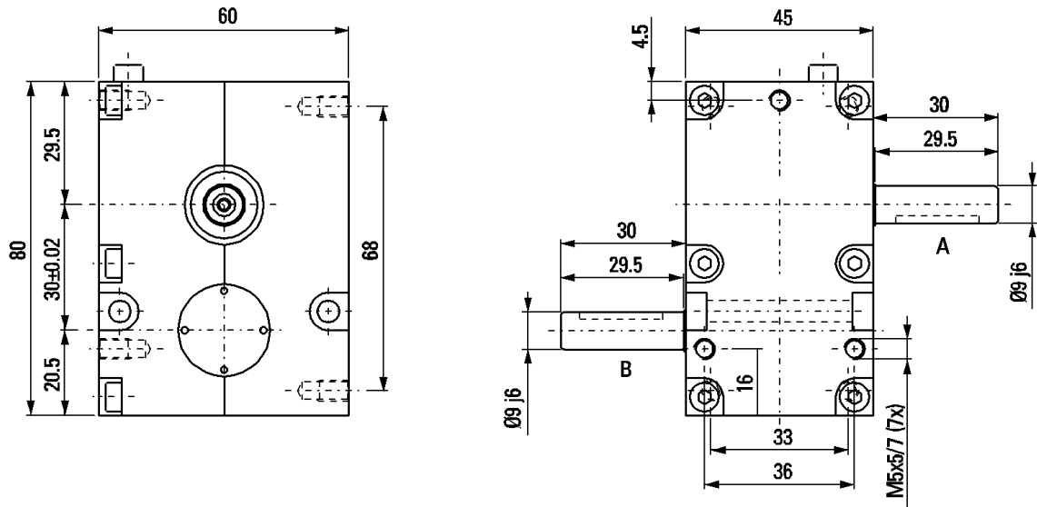
Abb. 11 Maßzeichnung XP 030
