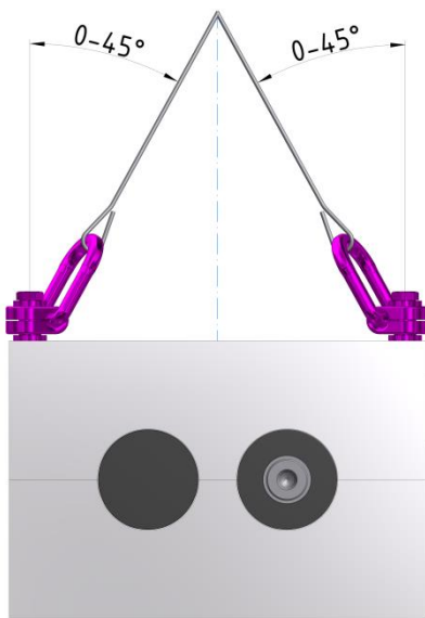
Abb. 29 Hebeanweisung
