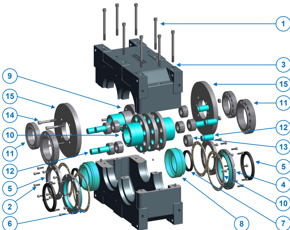
Abb. 37 Detail Montager Reihenfolge XP165-250
