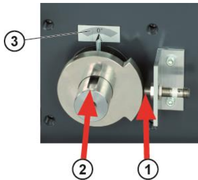
Abb. 32 Detail Positionsnocke
