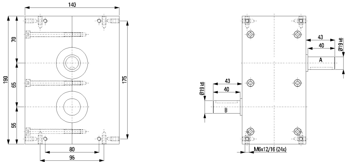
Abb. 14 Maßzeichnung XP 065
