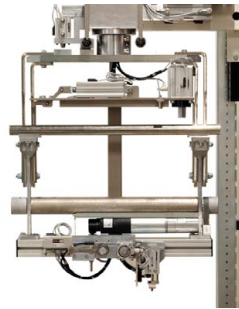
Verdeelmoduul Verteilermodul
