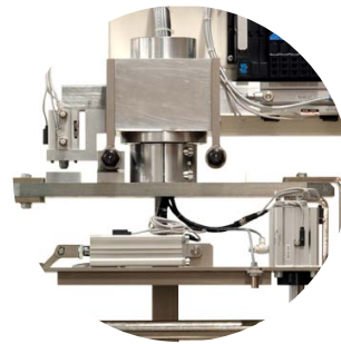
Aandrijfunit Antriebsunit
